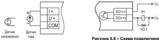
Рисунок 5.5 – Схемы подключения входных сигналов
